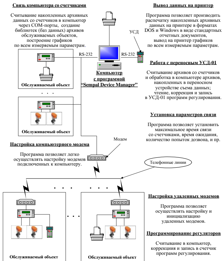
Рис.1. Основные функции программы "Sempal DM".
