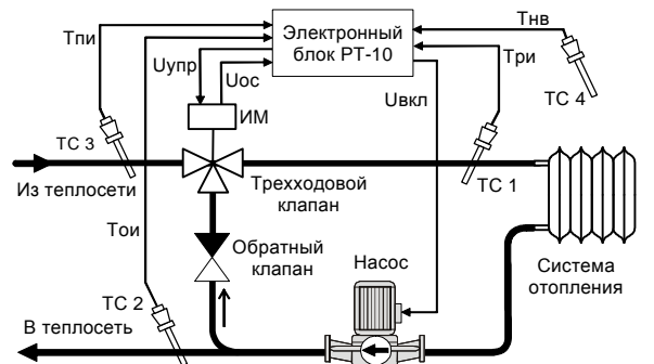
Рис.6 Регулирование температуры на выходе контура отопления с коррекцией по Тнв и управление циркуляционным насосом по температуре Тпи (конфигурация 5) .
