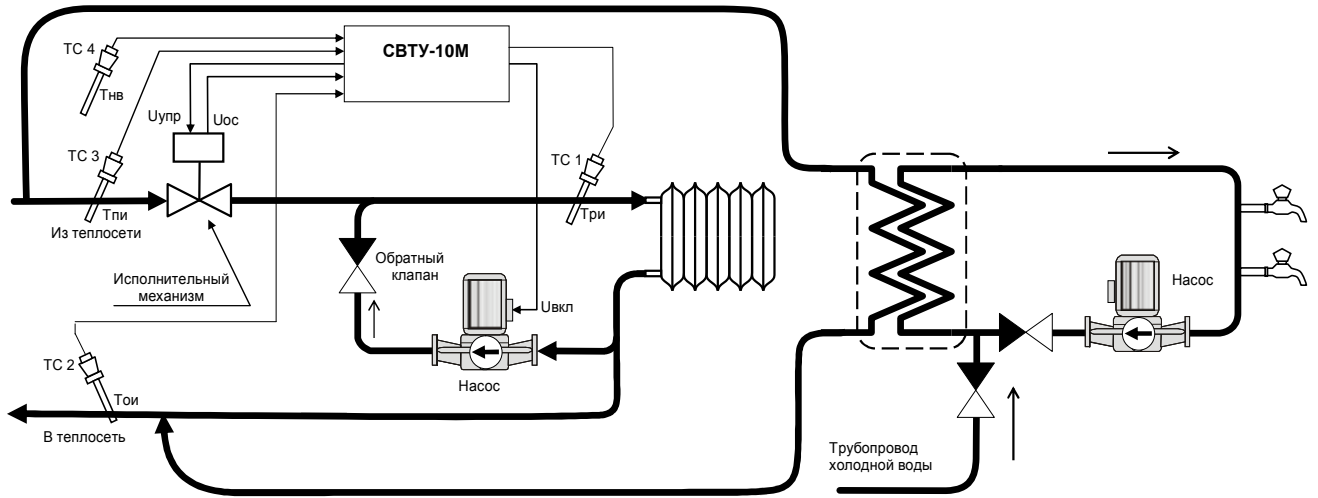
Рис. 9. Пример организации канала регулирования температуры отопления с использованием одноканального теплосчетчика СВТУ-10М в схеме с теплообменником.
