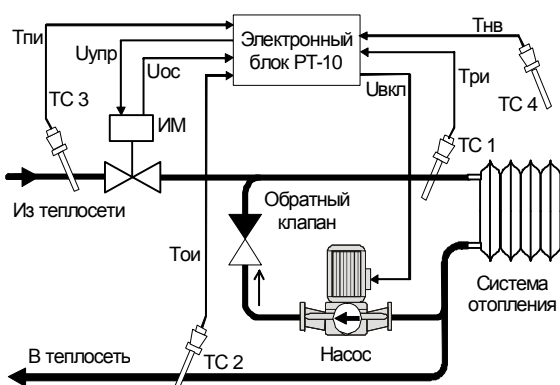
Рис.5 Регулирование температуры на входе контура отопления с ограничением температуры "обратки" и управление циркуляционным насосом (конфигурация 3) .
